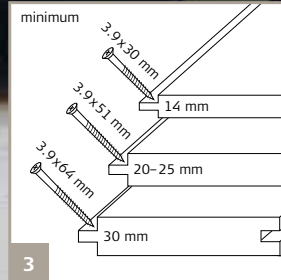
Skruer
