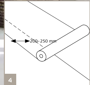
Dampspærre
