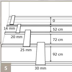
Strøfstande
