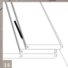
Sidste planke
